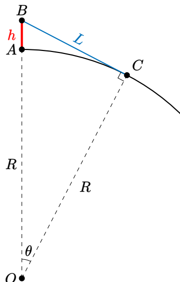
Figur 1: Siktlinjen BC tangerar jordytan i C .
