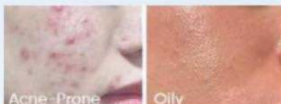
Acne-Prone
