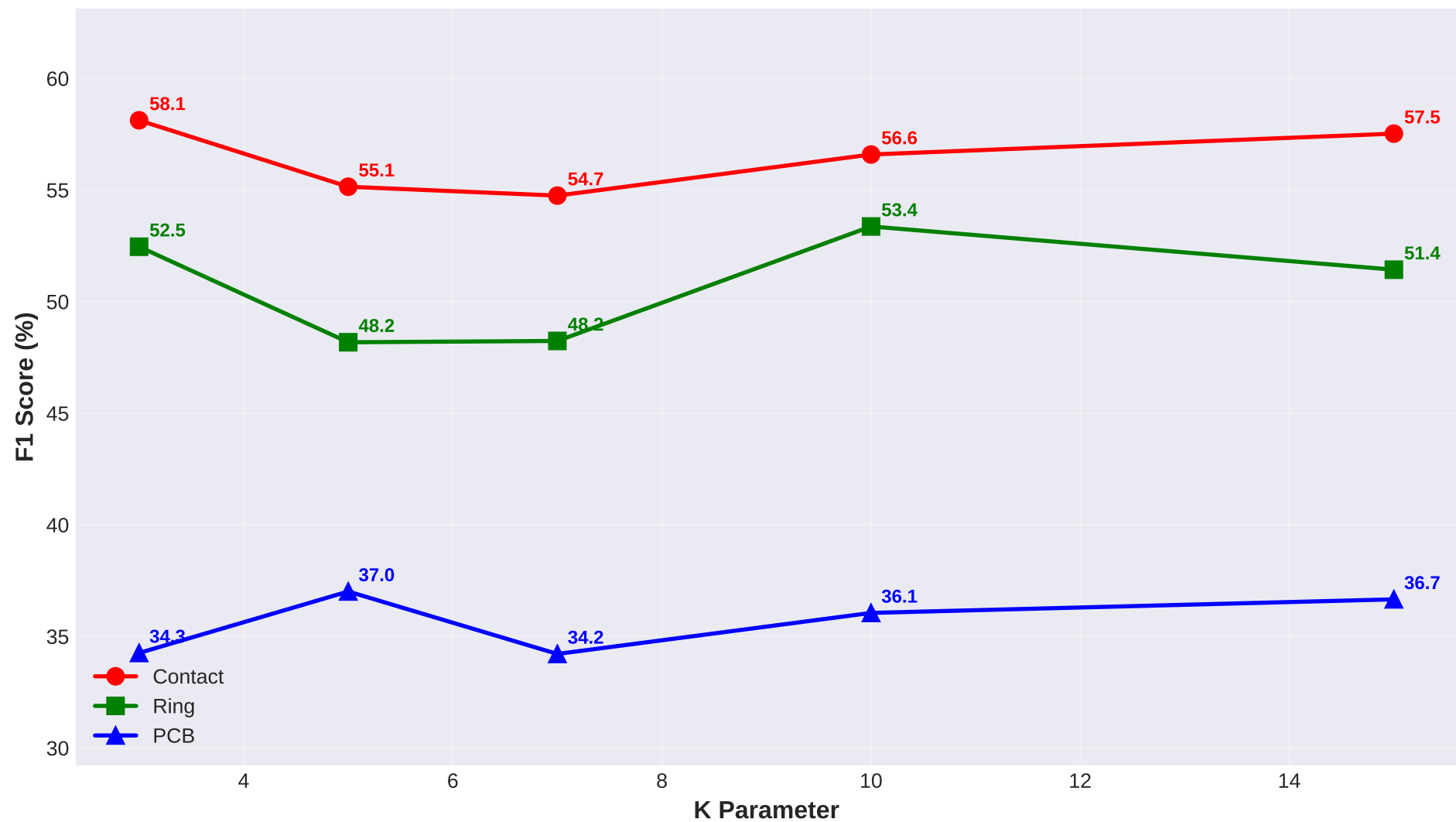
F1 Score vs K Parameter for Different Datasets
