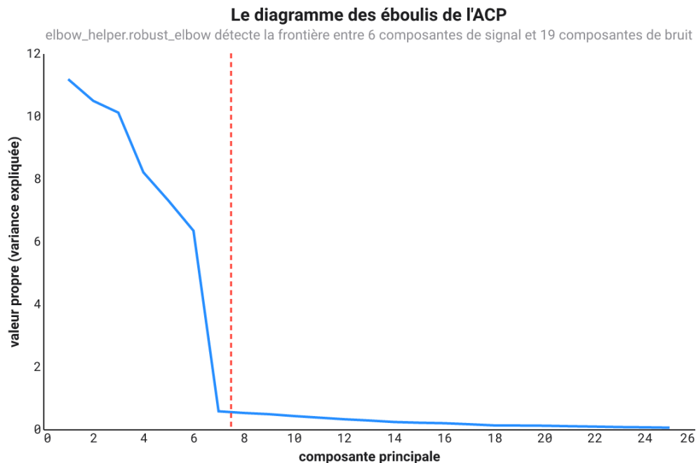
FIGURE 5 – Le diagramme des éboulis de l'ACP, avec le coude détecté par elbow_helper.robust_elbow (ligne rouge pointillée) à la frontière entre 6 composantes de signal et 19 composantes de bruit.
