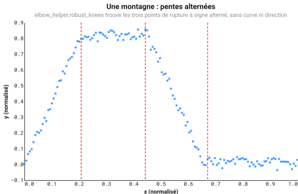
FIGURE 2 – Une courbe en montagne avec les trois points de rupture détectés par elbow_helper.robust_knees (lignes rouges pointillées) : montée, palier, descente, palier, retrouvés sans aucun argument curve ni direction .
