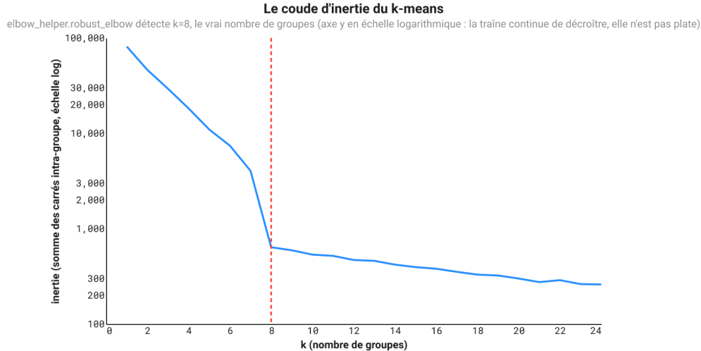
FIGURE 1 – La courbe d’inertie du k-means, axe y en échelle logarithmique, avec le coude détecté par elbow_helper.robust_elbow (ligne rouge pointillée) à k=8 , le vrai nombre de groupes, et une traîne qui continue de décroître doucement au-delà.
