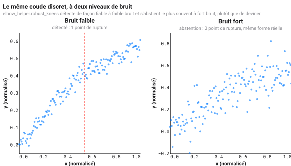
FIGURE 4 – Le même coude discret à deux niveaux de bruit : à faible bruit (gauche), détecté avec un point de rupture ; à fort bruit (droite), abstention avec zéro point de rupture, la même forme réelle sous les deux panneaux.
