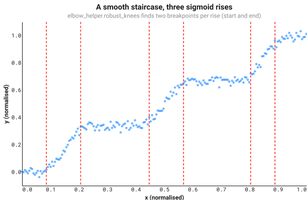
FIGURE 3 – Un escalier lisse construit à partir de trois sigmoïdes logistiques, avec les six points de rupture détectés par elbow_helper.robust_knees (lignes rouges pointillées) encadrant chacun le début et la fin d’une montée.
