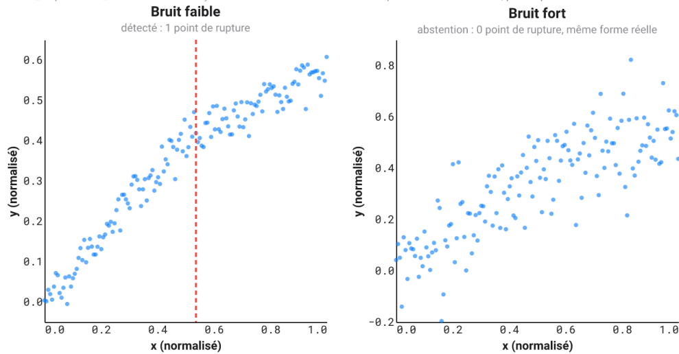
FIGURE 4 – Le même coude discret à deux niveaux de bruit : à faible bruit (gauche), détecté avec un point de rupture ; à fort bruit (droite), abstention avec zéro point de rupture, la même forme réelle sous les deux panneaux.
