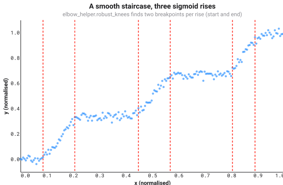
FIGURE 3 – Un escalier lisse construit à partir de trois sigmoïdes logistiques, avec les six points de rupture détectés par elbow_helper.robust_knees (lignes rouges pointillées) encadrant chacun le début et la fin d’une montée.
