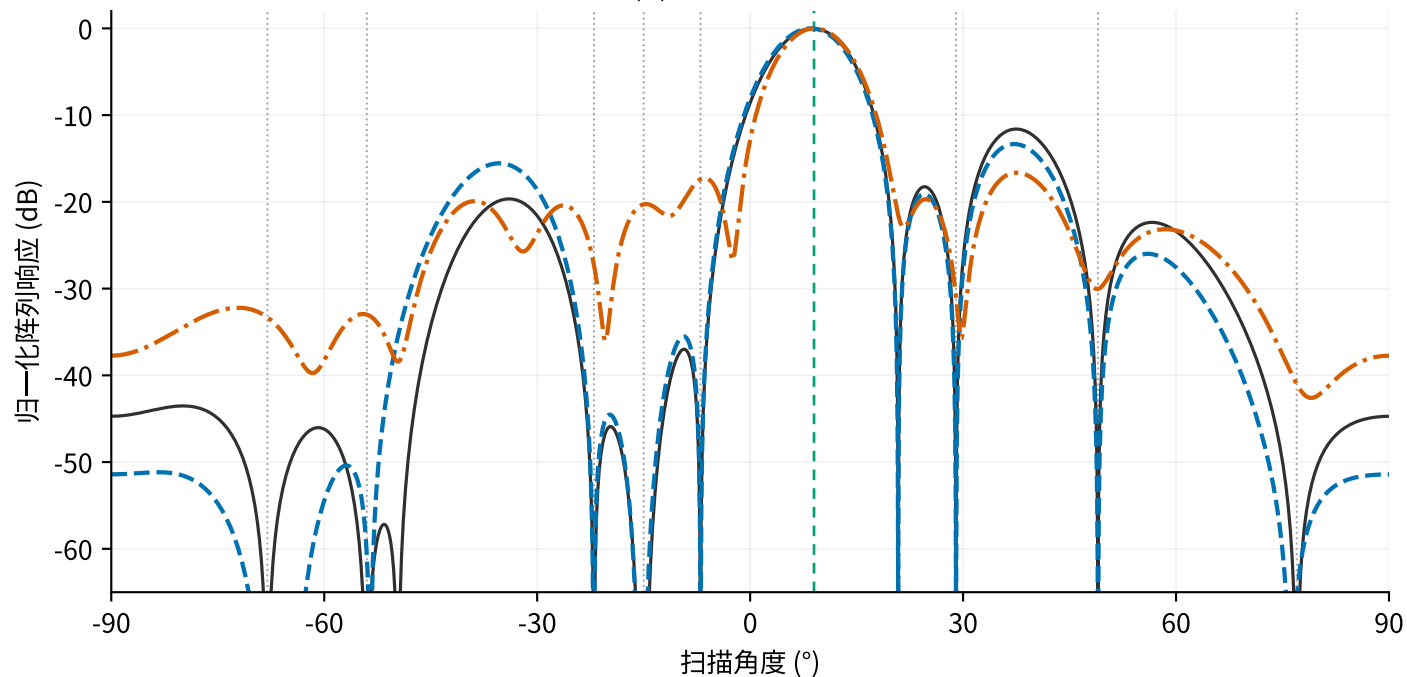
(a) 全角域方向图
