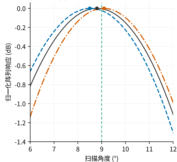
(b) 期望方向附近的局部峰
