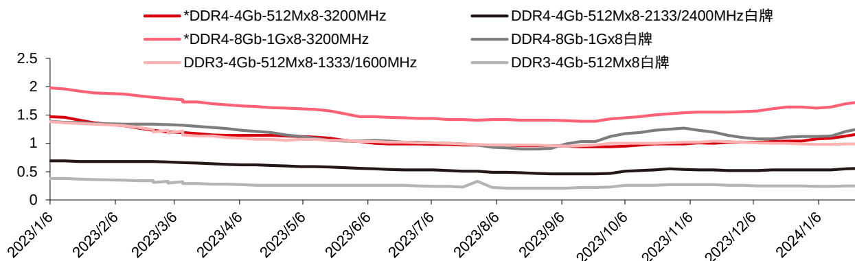
图 2: DRAM 周度价格（美元）
