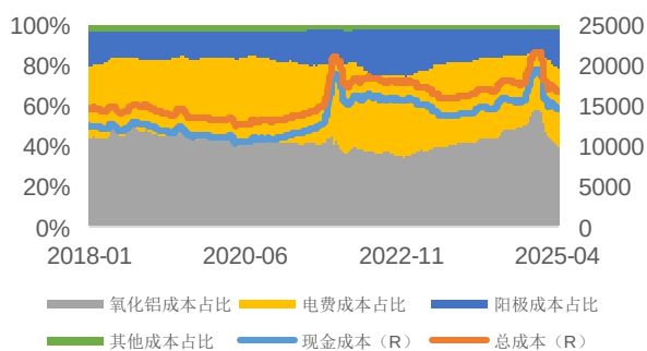
图表 63：中国电解铝成本结构（元/吨）
