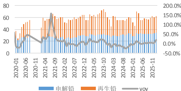
图表 32：中国精炼铅产量（万吨）
