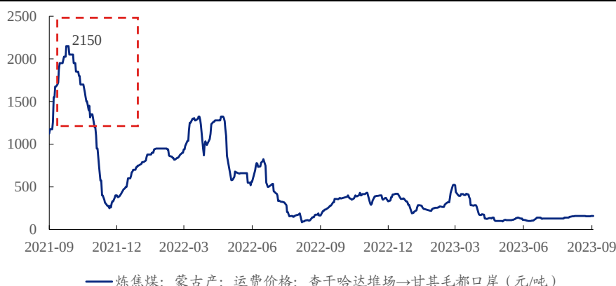
图表 47、查干哈达至甘其毛都短盘运费波动较大
