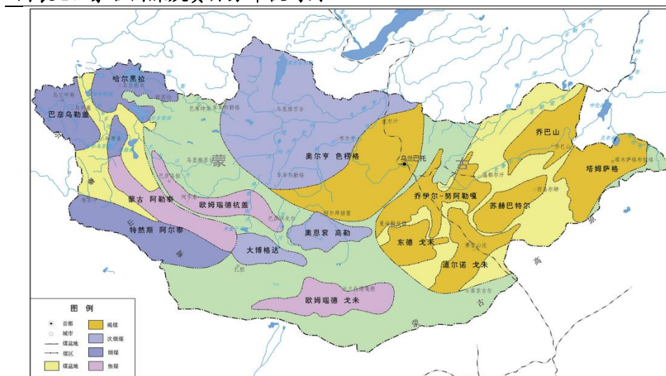
图表 1、蒙古国煤炭资源分布较均衡
