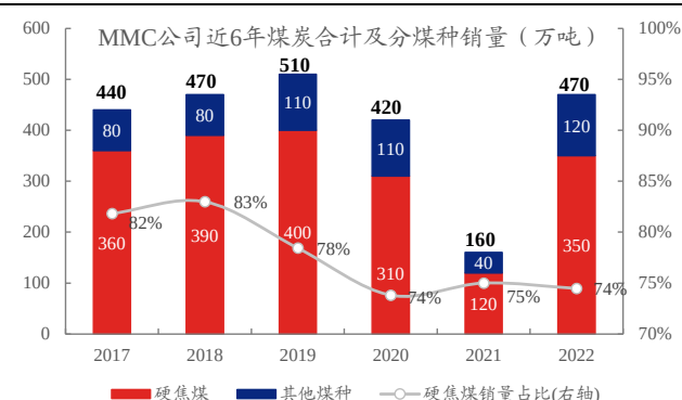
图表 24、MMC 公司煤炭销售以硬焦煤为主
