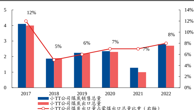
图表 31、2022 年小 TT 公司煤炭出口量占全蒙 8%（百万吨）
