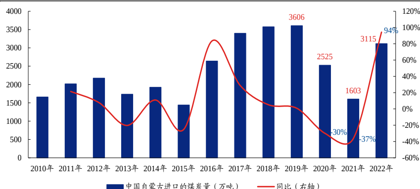
图表 39、2022 年中国进口的蒙煤量仍未达历史峰值
