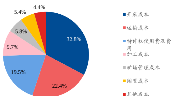
图表 26、2022 年 MMC 公司吨煤成本为 54.3 美元
