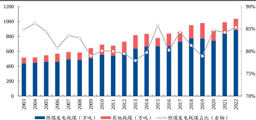
图表 11、蒙古国煤炭消费以燃煤发电为主，占比超过 80%
