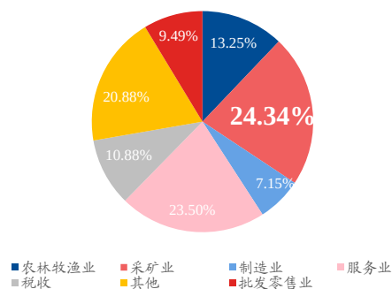
图表 5、2022 年蒙古国采矿业占 GDP 接近 1/4
