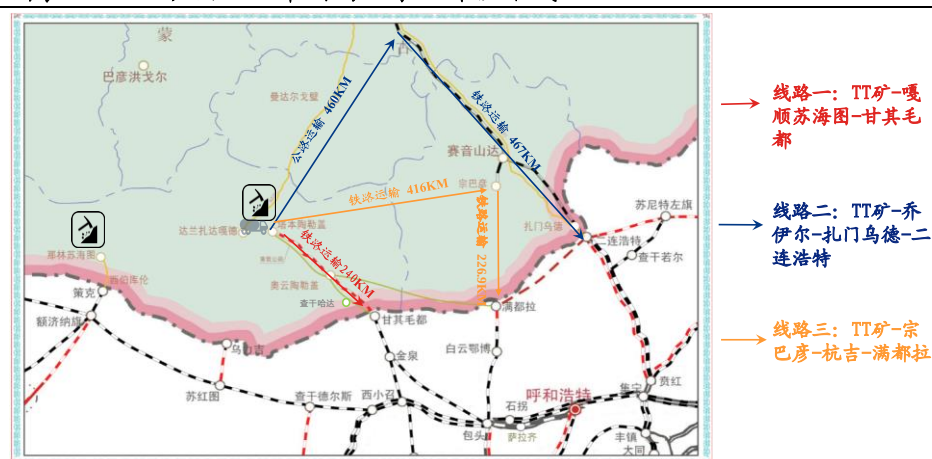
图表 13、TT 矿出口至中国的 3 条运煤铁路线
