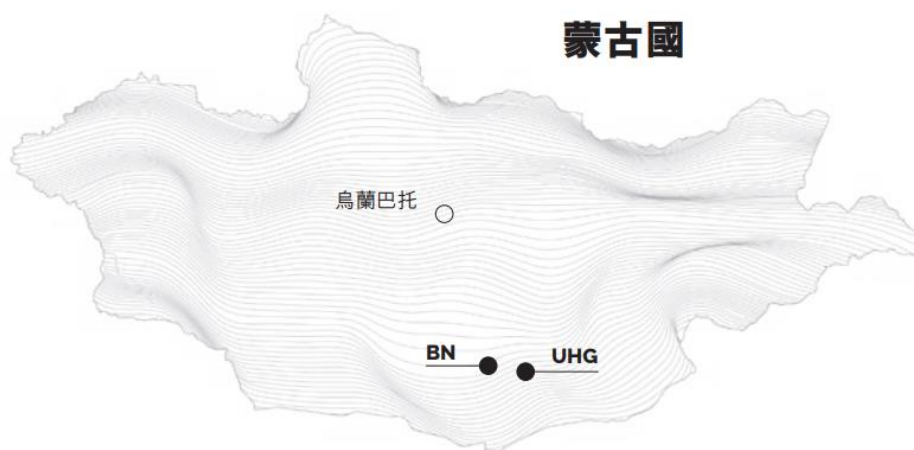
图表 21、MMC 公司主要煤炭产地——UHG 和 BN
