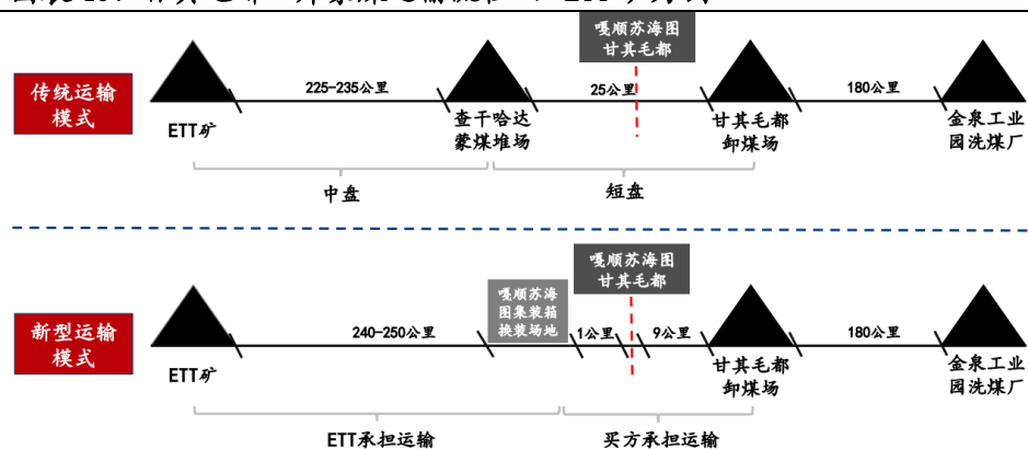
图表 46、甘其毛都口岸蒙煤运输流程-以 ETT 矿为例
