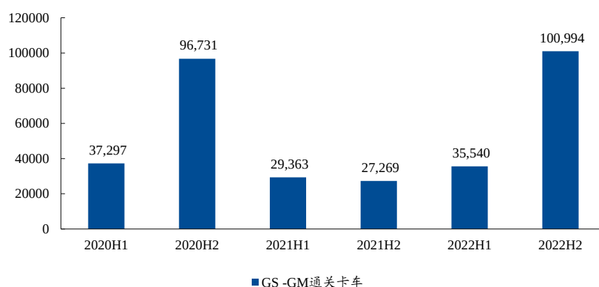
图表 25、MMC 公司通过 GS-GM 的车辆数于 2022H2 明显回升 (辆)
