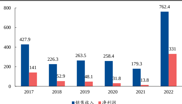
图表 30、小 TT 公司销售收入及净利润（十亿图格里克）
