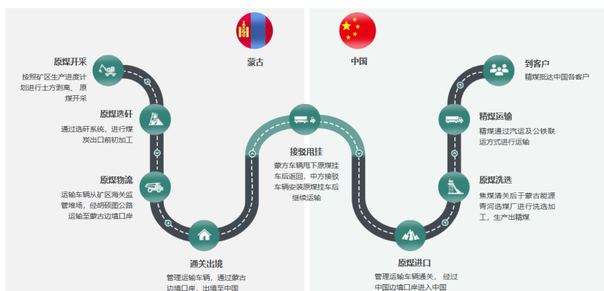
图表 35、蒙古能源煤炭生产主要销往中国新疆
