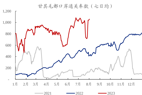
图表 52、甘其毛都口岸通关车数（辆）
