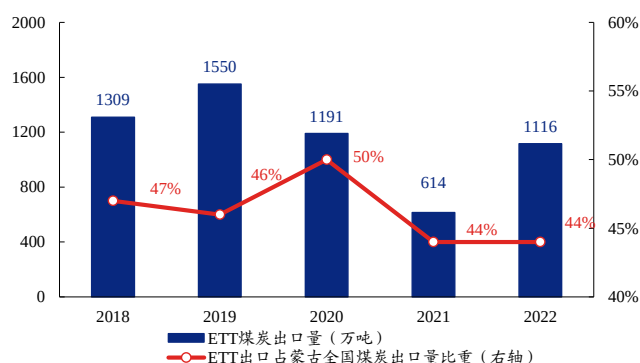
图表 19、2022 年 ETT 公司煤炭出口占全蒙比重为 44%
