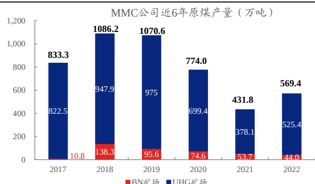
图表 23、2022 年 MMC 公司原煤产量较高峰期下滑 47.6%
