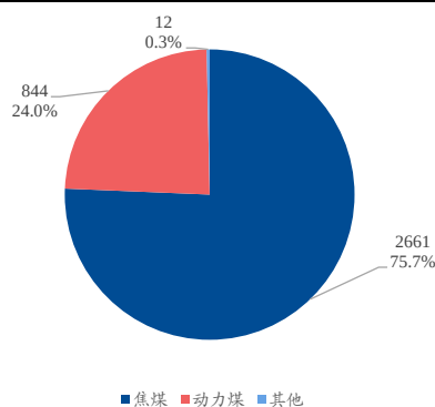
图表 41、2023 年 1-7 月蒙煤进口结构 (万吨)
