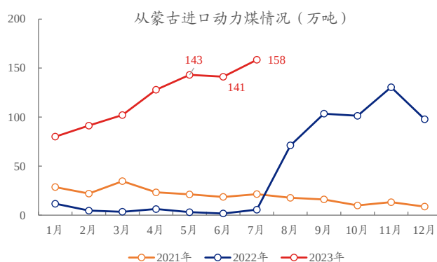
图表 43、中国自蒙古进口的动力煤量
