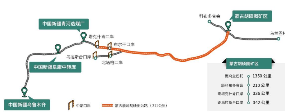
图表 36、蒙古能源胡硕图矿区距中国塔克什肯口岸约 336 公里
