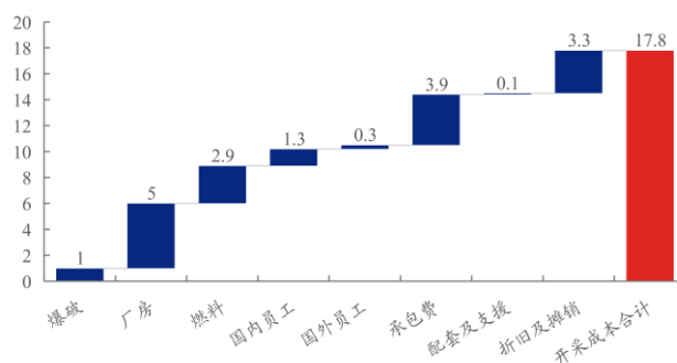
图表 27、2022 年 MMC 吨煤开采成本为 17.8 美元
