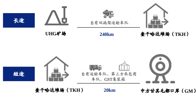
图表 28、MMC 公司煤炭运至到中国甘其毛都口岸需经两段运输
