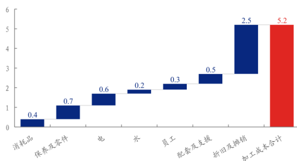
图表 29、2022 年 MMC 公司吨煤加工成本为 5.2 美元
