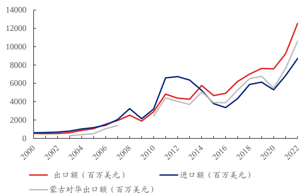
图表 6、蒙古国历年进出口额
