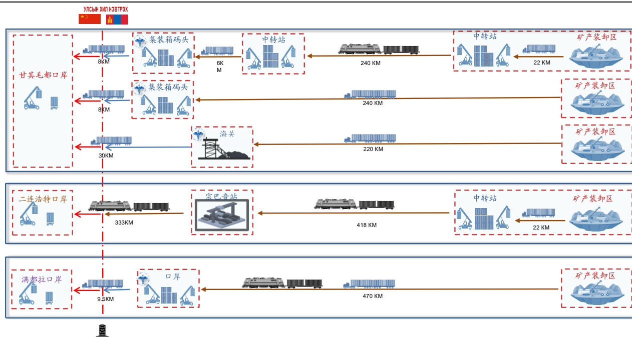
图表 32、小 TT 公司计划拓展其他口岸的煤炭出口
