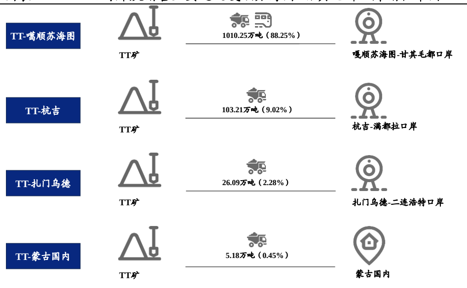
图表 20、ETT 公司煤炭销售主要通过嘎顺苏海图-甘其毛都口岸销往中国
