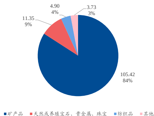
图表 7、2022 年蒙古国出口商品结构 (亿美元)
