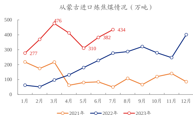
图表 42、中国自蒙古进口的焦煤量
