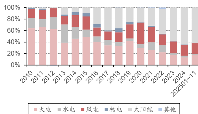
图 3：国内各类电源新增发电设备容量结构
