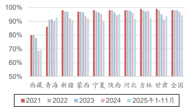
图 9：各地区光伏并网利用率
