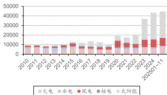
图 2：国内各类电源新增发电设备容量（万 kW）
