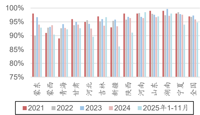
图 8：各地区风电并网利用率
