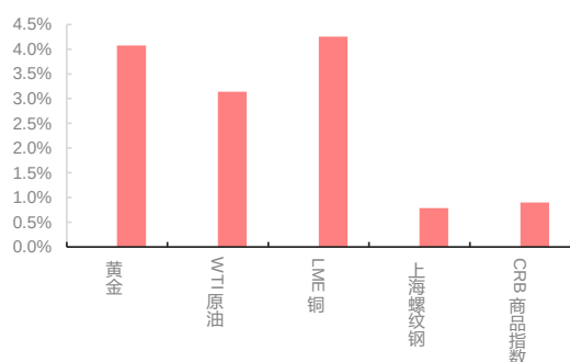
图 7: 商品表现
