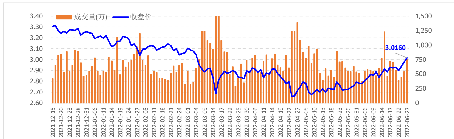
图2 SH300ETF走势图
