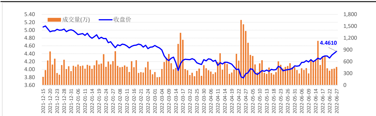
图3: SZ300ETF走势图
