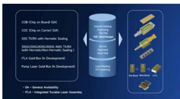
图37. BOX 器件封装技术平台/高速光引擎产品解决方案 图38. 相干光学技术平台/FAU 无源光器件产品解决方案
