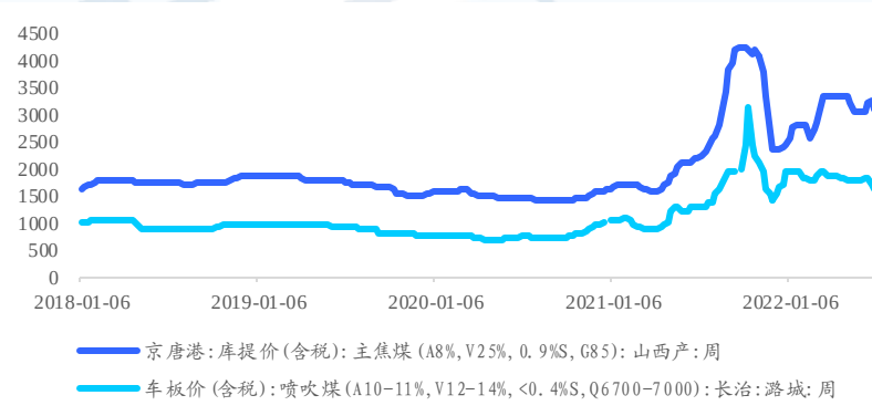
图 23：2018年以来无烟粉煤和主焦煤港口价整体走势一致
