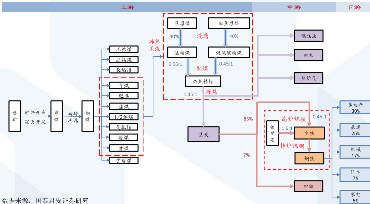
图1：煤焦钢产业链情况
