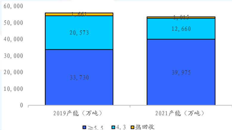
图13：不同碳化室高度焦炭产能
