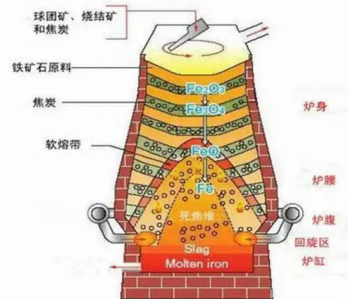
图26：高炉炼铁流程
