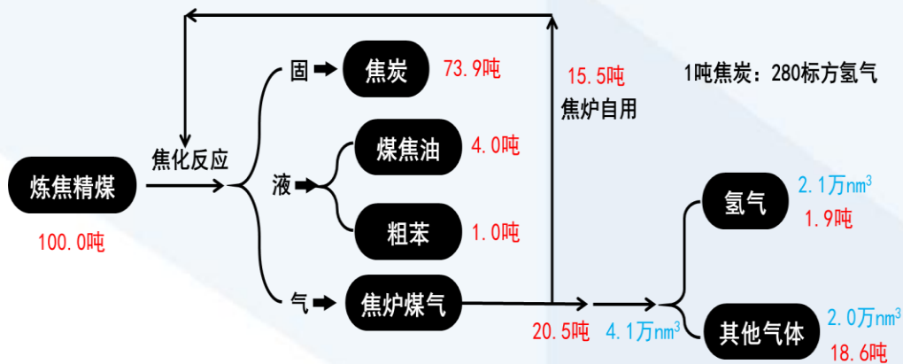
图18：焦化副产氢流程
