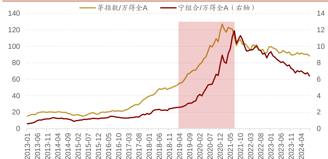
图 25：主动偏股基金重仓的茅指数、宁组合显著跑赢万得全 A
