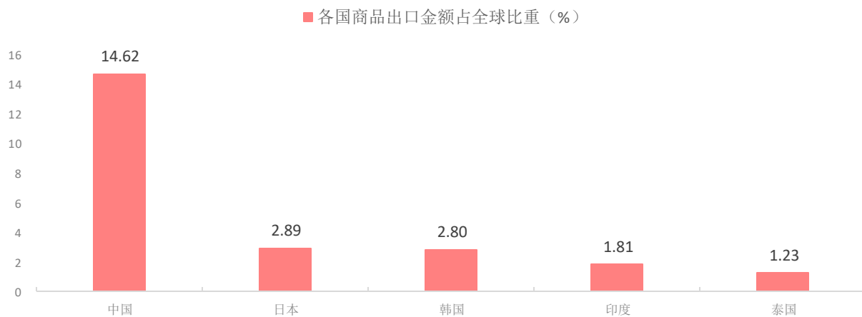
图 7: 亚洲主要经济体出口占全球份额
