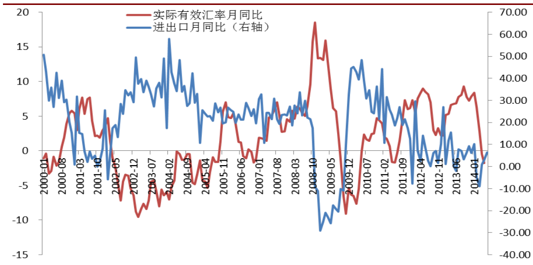
图 2：中国进出口月同比与实际有效汇率月同比
