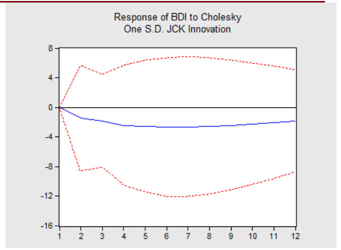
图 5：BDI 指标对进出口指标的脉冲响应
