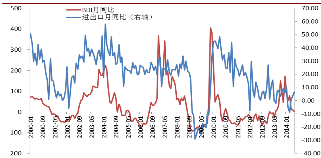
图 1：BDI 指数月同比领先中国进出口增速约三个月
