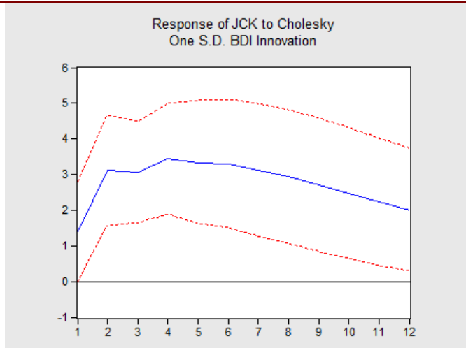
图 4：进出口指标对 BDI 指标的脉冲响应
