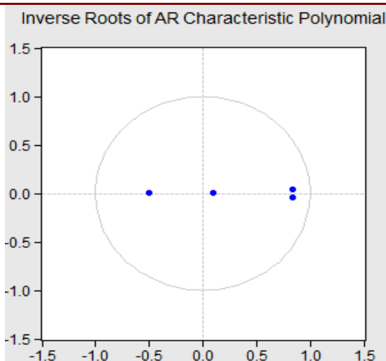
图 3：AR 根检验结果
