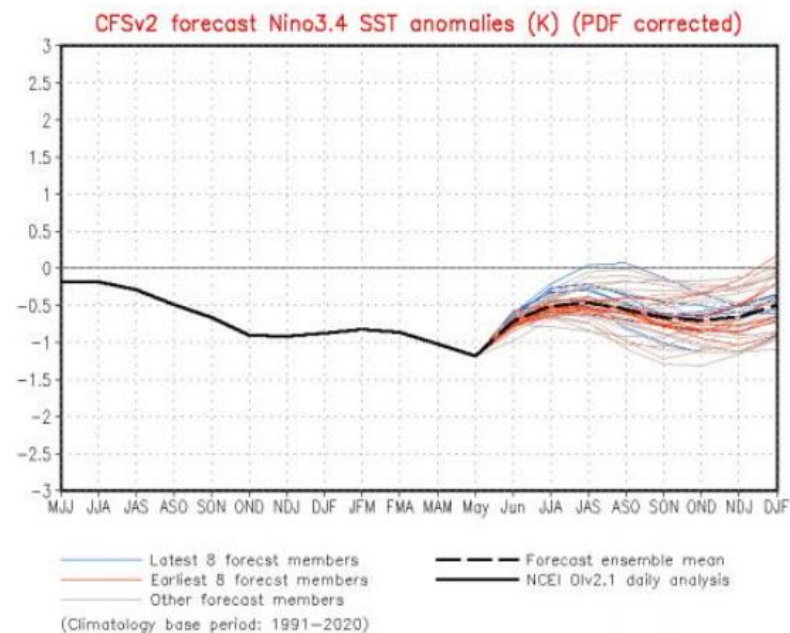
图27：拉尼娜预测
