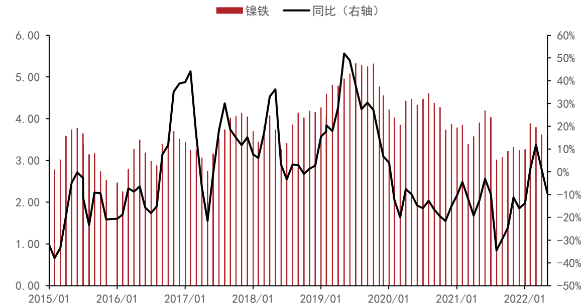
图14：镍铁产量（万吨）
