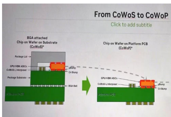
图 7: CoWoS 与 CoWoP 对比
