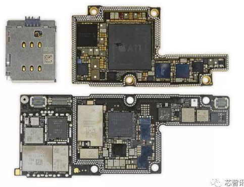
图 8: iPhoneX 主板拆解
