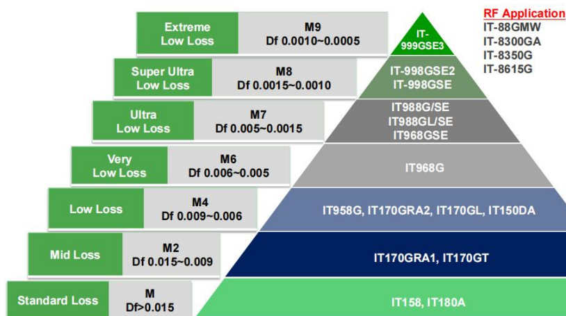
图 10：联茂电子 M1-M9 覆铜板材料
