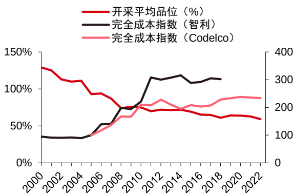
图 34：智利采出矿石铜品位以及完全成本情况
