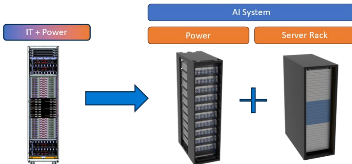
图表24: Meta 与微软共同推出 Mt. Diablo 400 供电方案, 主要思路是单设电源机柜和 400V 供电
