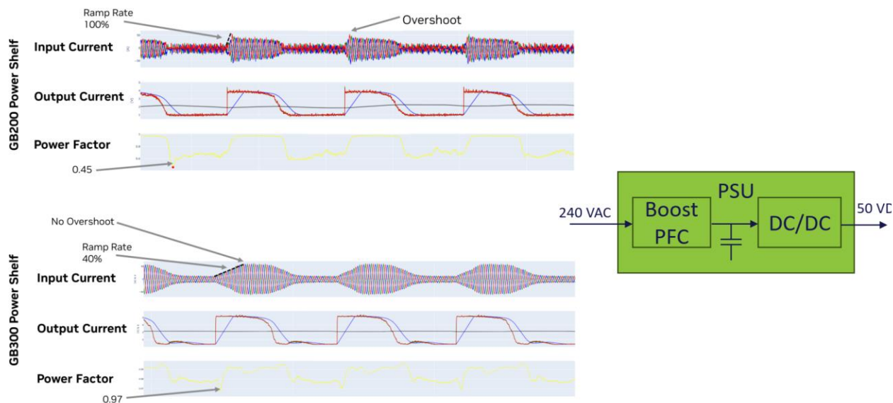
图表50：通过在输入级使用 Boost 电路，GB300 Power Shelf 电能质量较 GB200 的有显著提升
