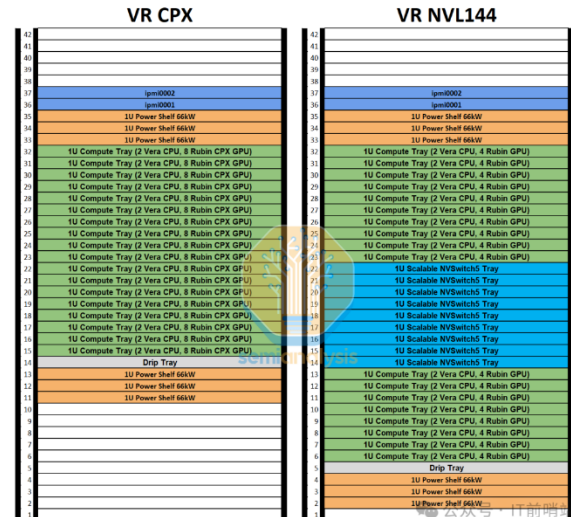
图表43: Rubin 芯片的 NVL144 机柜升级到 66kW Power Shelf
