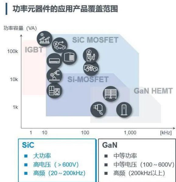
图表52： SiC 可用于大功率高压场合，GaN 则用于中等功率、中等电压、高频场合
