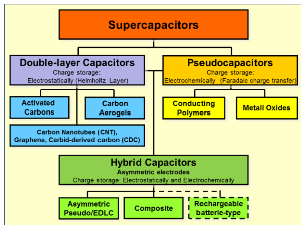
图表66： 超级电容器按原理可分为三类
