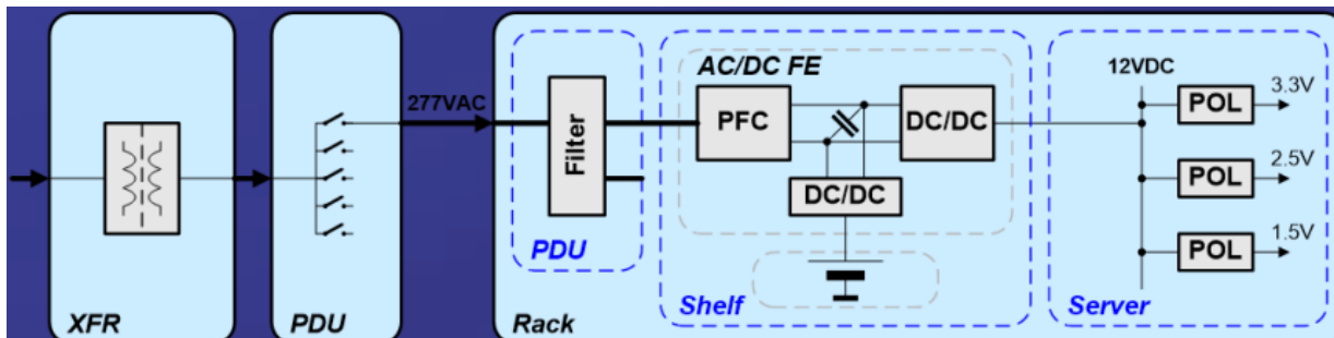
图表18: ORV2 升级到 6.6kW Powershell, 改用锂电池 BBU, 但输出电压仍为 12V
