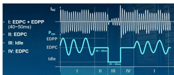
图表61： 配备 CBU 前，GPU 负荷波动影响交流输入电流一起波动
