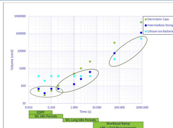
图表83: 电容适合毫秒级波动, 电池适合秒级以上波动
