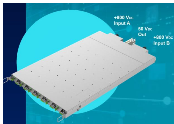
图表57： 台达 800V/50V DC/DC 机柜级电源
