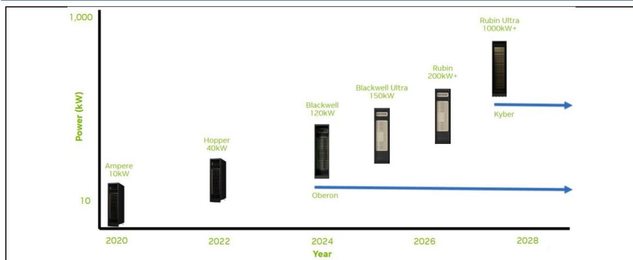
图表5： 随着 GPU 功率提升，单机柜功率已提升至 MW 级别
