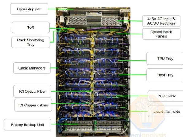
图表8：谷歌 TPU 机柜内含 AC/DC 电源模块
