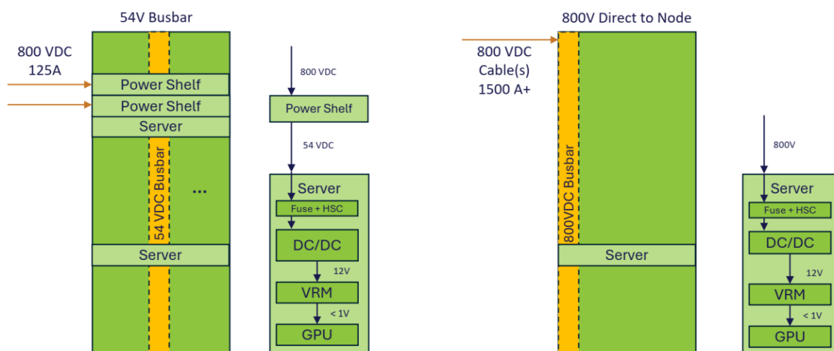
图表54： 英伟达 800V MGX 机柜内增设 800 转 54V/12VDC/DC 环节
