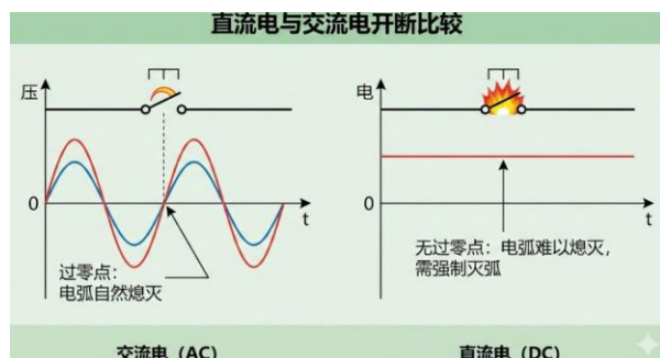
图表74： 直流电较交流电更难开断
