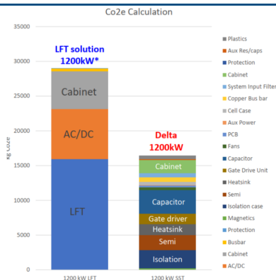
图表34： SST 较多使用半导体、电容器等电子元器件，较线性变压器大大减少了碳排放
