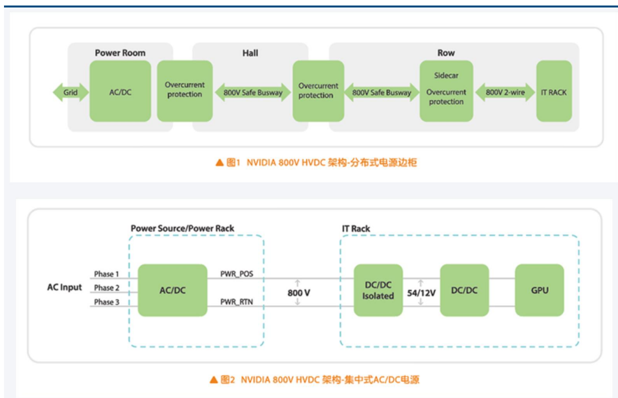
图表36： 英伟达 800V 数据中心配电系统结构示意图
