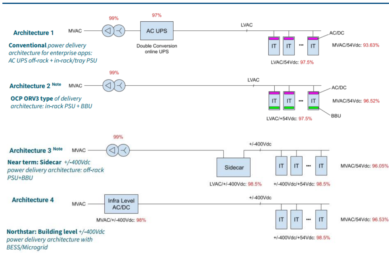
图表14： 通过内置 BBU、采用边柜供电、采用±400V 高压直流供电等方式，效率可以提升到 96%以上
