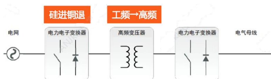
图表16: SST 关键技术主要在电力电子变换器和高频隔离变压器
