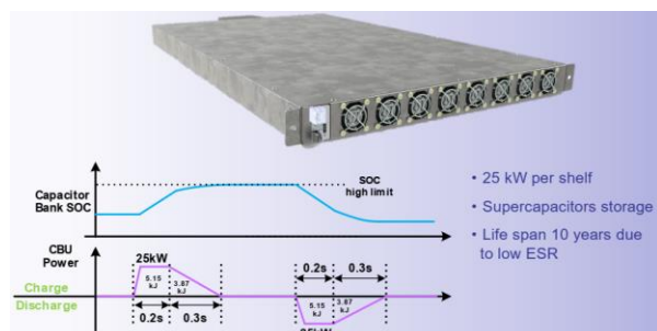
图表63： 台达推出的 25kW CBU，内含超级电容器
