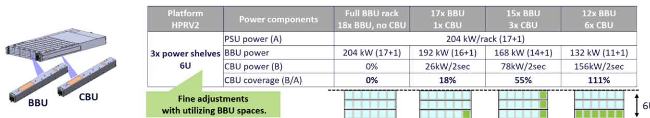
图表65： CBU 可以部分取代 BBU
