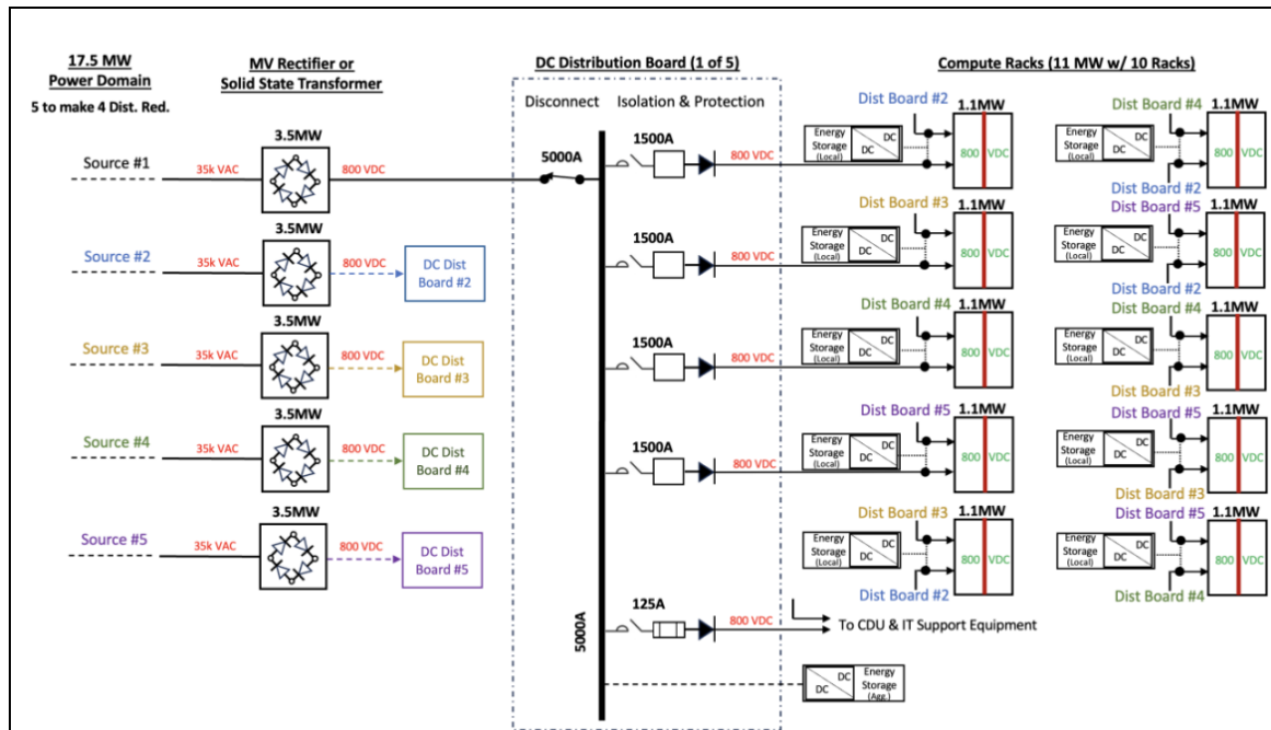
图表76： 英伟达 800V 参考设计中明确提出使用 1500A 固态断路器
