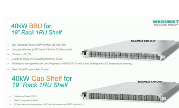
图表73： 麦格米特推出了 40kWBBU 和 CBU 产品
