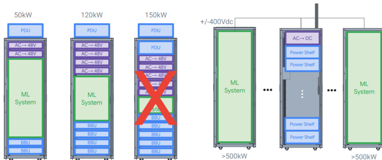
图表13： 传统交流供电方案（左）因为占用空间过大而不可接受，通过直流供电和电源外置（右）得以解决
