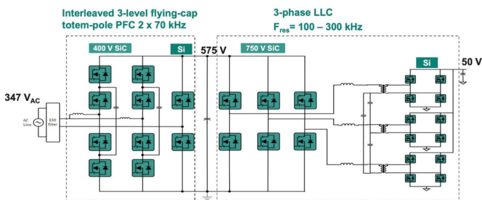
图表47： 第二代 AI PSU 主要采用三电平拓扑取代两电平
