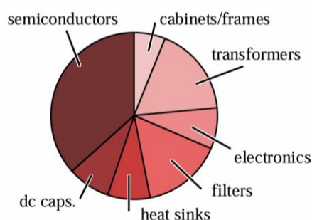
图表33: SST 成本构成中半导体功率器件、高频变压器占前两位
