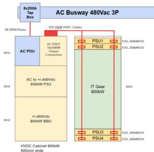
图表22： HPR V4 方案通过采用 \pm 400\text{V HVDC} ，支持机柜功率达到 800kW
