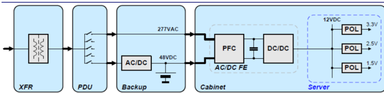
图表17： ORV1 使用直流 12V 输出和 4.2kW Powershelf，单机柜功率不超过 12.6kW
