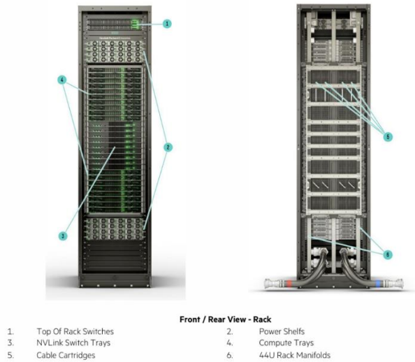
图表42: NVL72 含有 8 个 33kW Power Shelf
