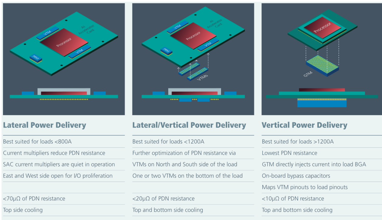
图表59： GPU 周边电源由外周布局向垂直供电迭代
