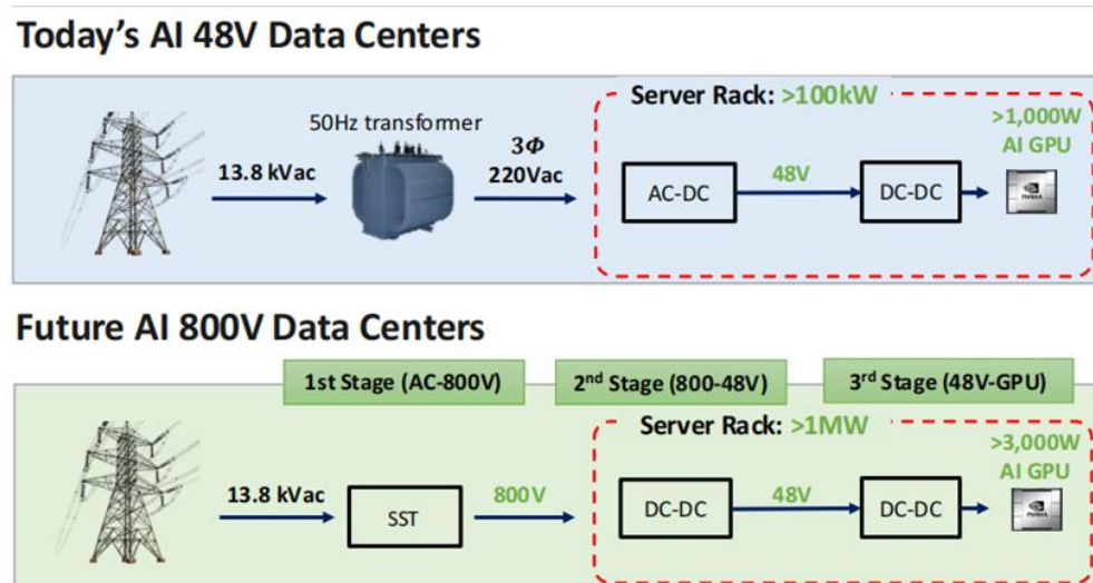
图表15: SST 直接将 13.8kV 交流电转换为 800V 直流电, 节省一级变压器
