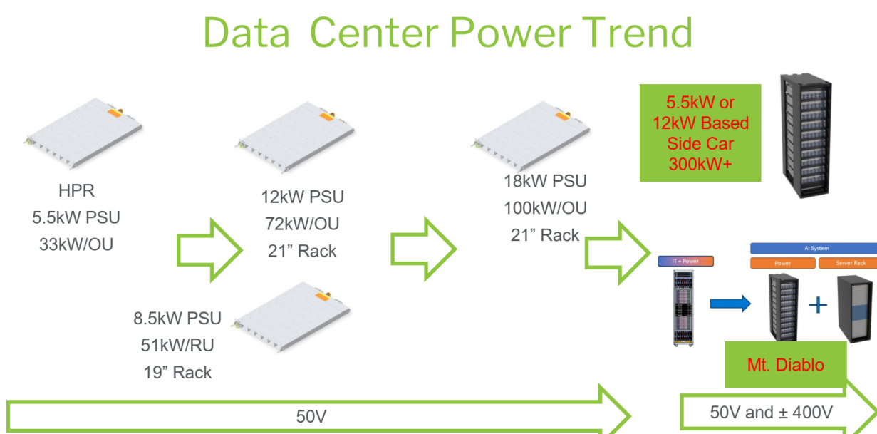
图表41： PSU 功率不断提升
