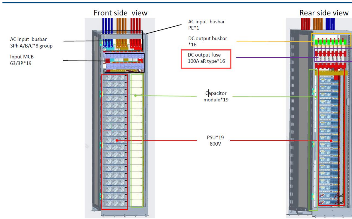
图表81：熔断器安装在 HVDC 电源机柜内部
