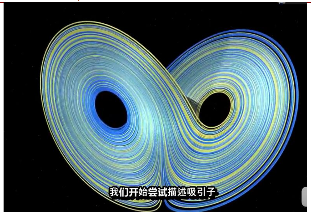
图 4：洛伦兹方程组解的几何示意图
