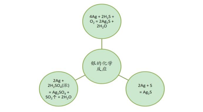
图 73 银的化学反应
