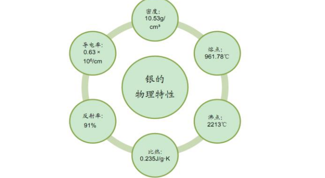
图 72 银的物理性质
