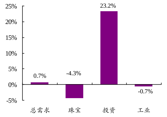
图 16：2000-2010 复合增长率
