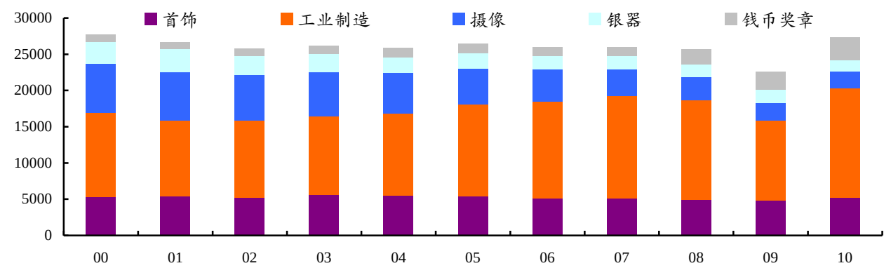
图 52：白银需求（吨）
