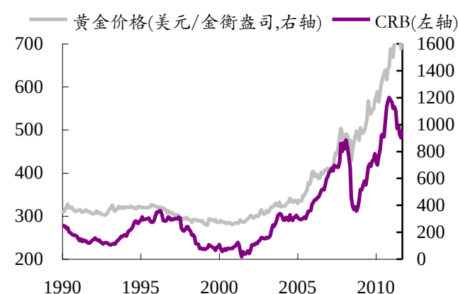
图 40：金价与 CRB
