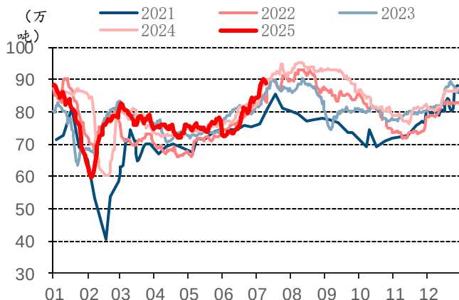
图 21: 沿海六大电厂日耗
