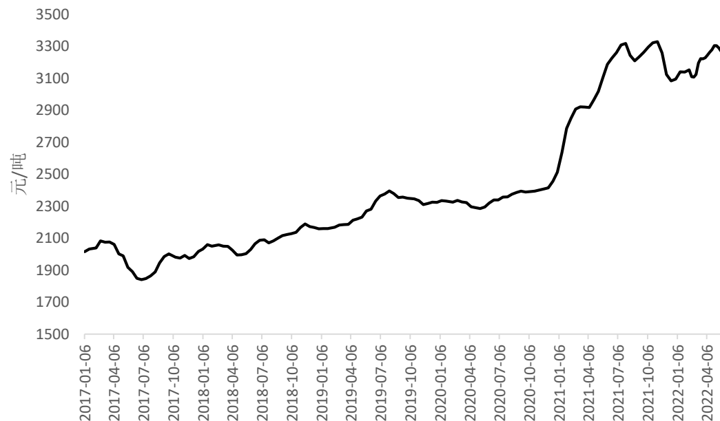
图3.5：铁水成本（64家钢厂）（元/吨）
