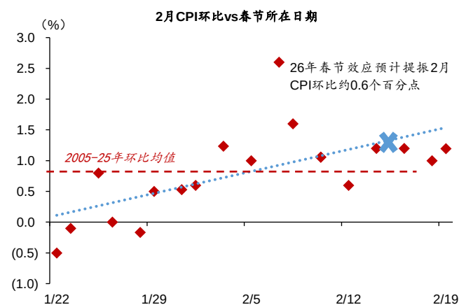
图表4：根据我们估算，春节效应或提振2月CPI环比约0.6个百分点
