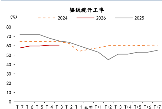
图表15: 铝线缆开工率环比上行, 低于往年同期
