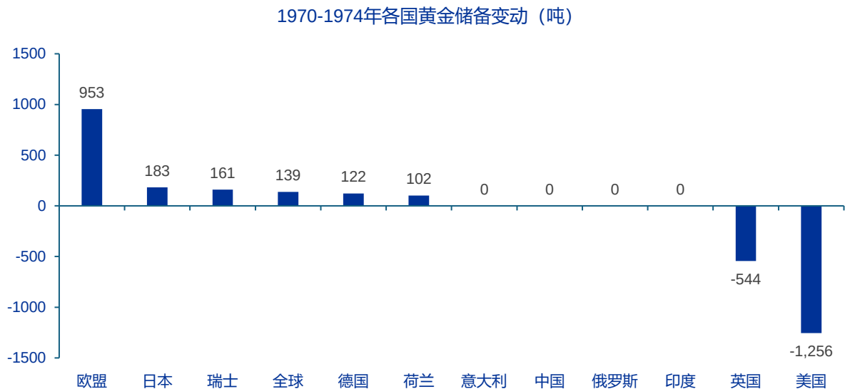
图 29：全球央行持续购金并且避险需求大幅上升
