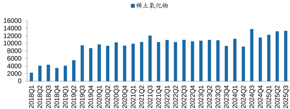
图74： 2018年以来美国Mount Pass季度稀土产量（吨）
