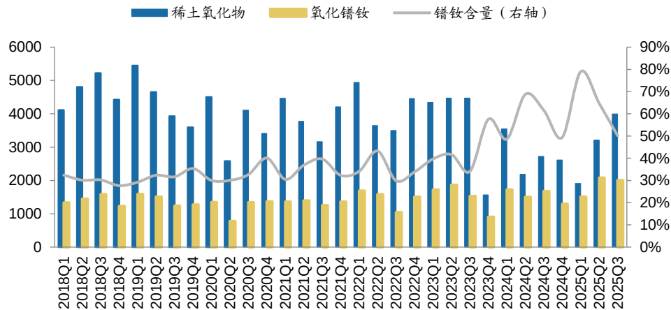
图75： 2018年以来澳大利亚莱纳斯季度稀土产量（吨）
