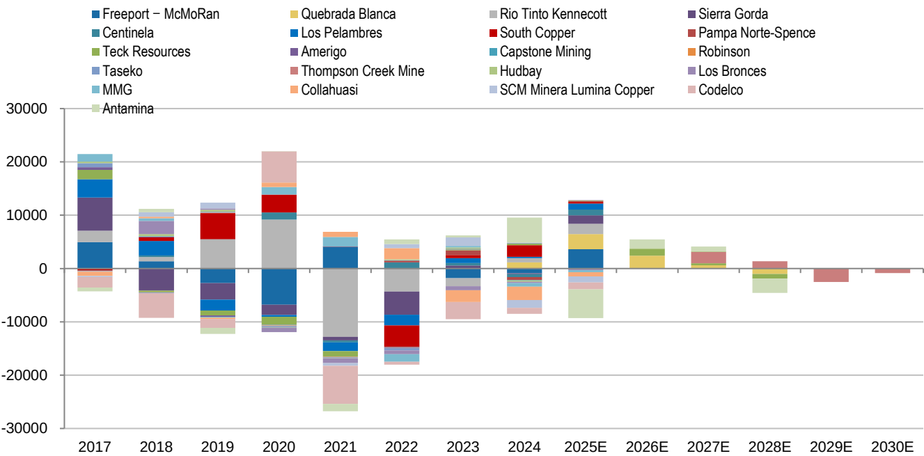
图78：海外主要公司每年钼矿产量Δ（吨）
