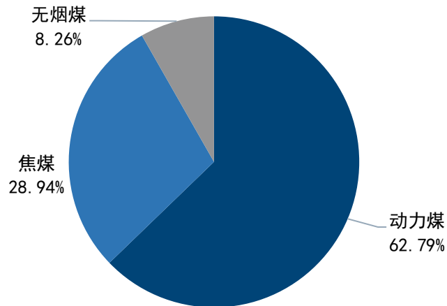
图11：2022年分煤种产量占比情况
