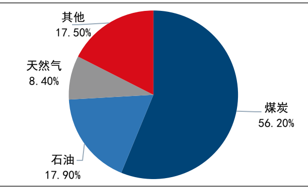
图10：2022年能源消费构成
