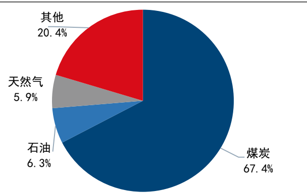
图9：2022年一次性能源生产占比
