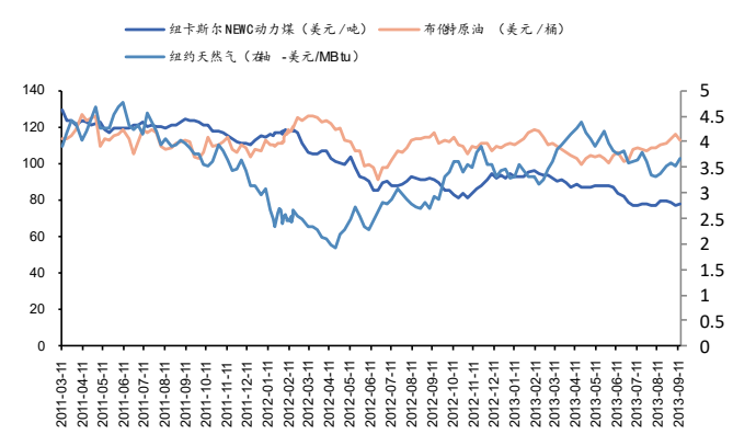
图表4:2011 年能源价格没有大幅上涨
