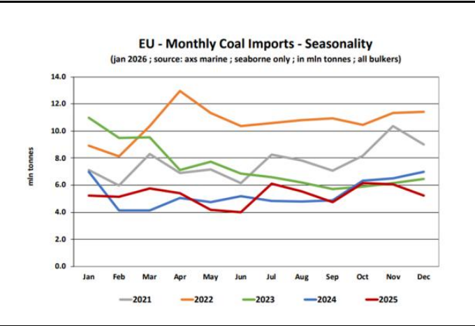
图表9:欧盟煤炭进口月度变化（百万吨）
