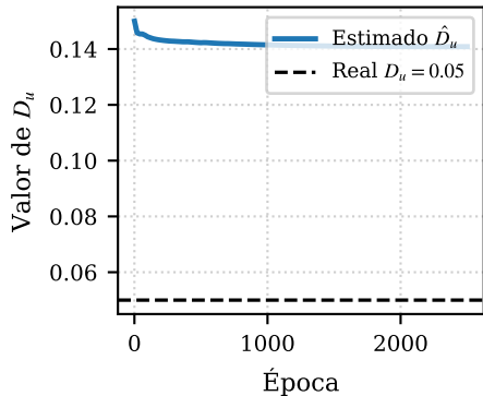
(a) Difusividade Ativador \hat{D}_u
