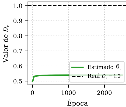
(b) Difusividade Inibidor \hat{D}_v
