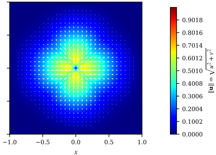
(b) \|\mathbf{u}\| em t=0,5\text{ s}
