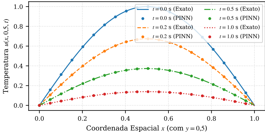
Perfil Transversal Térmico: Solução Exata vs PINN
