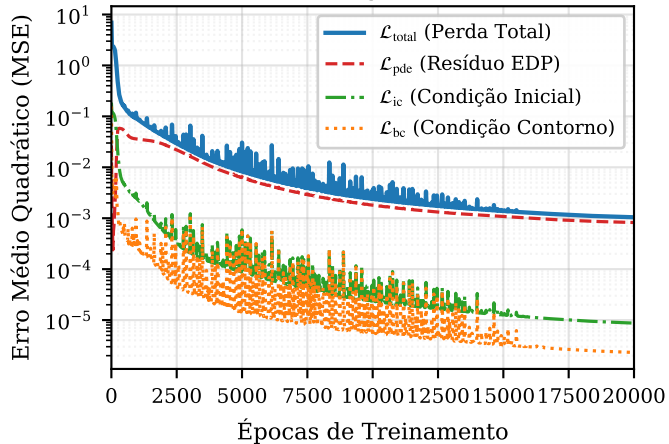
(b) Equação de Burgers 2D ( \nu = 0,01 \text{ m}^2/\text{s} )
