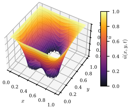
(b) Relevô Térmico 3D ( t = 2,0\text{ s} )
