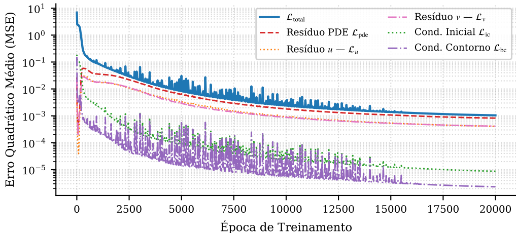
Convergência das Perdas — Burgers 2D ( \nu = 0.01 , 20.000 épocas)
