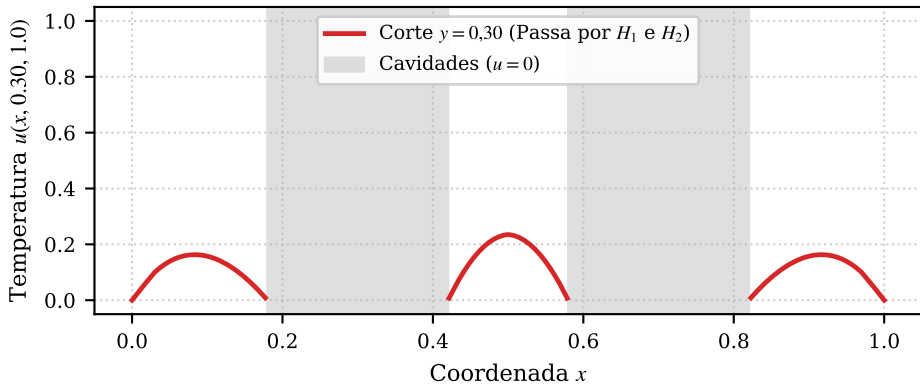
Perfil Unidimensional de Temperatura em t = 1.0 \backslash s
