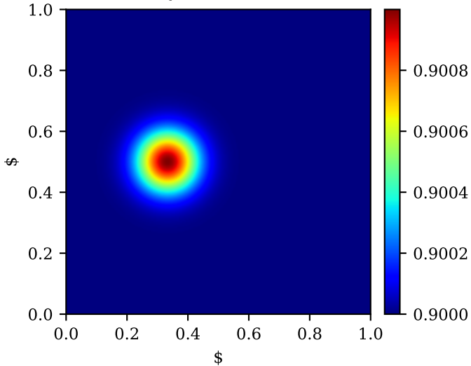
(a) Condição Inicial Exata (x,y,0)$ (Perturbação Gaussiana \varepsilon = 10^{-3} )
