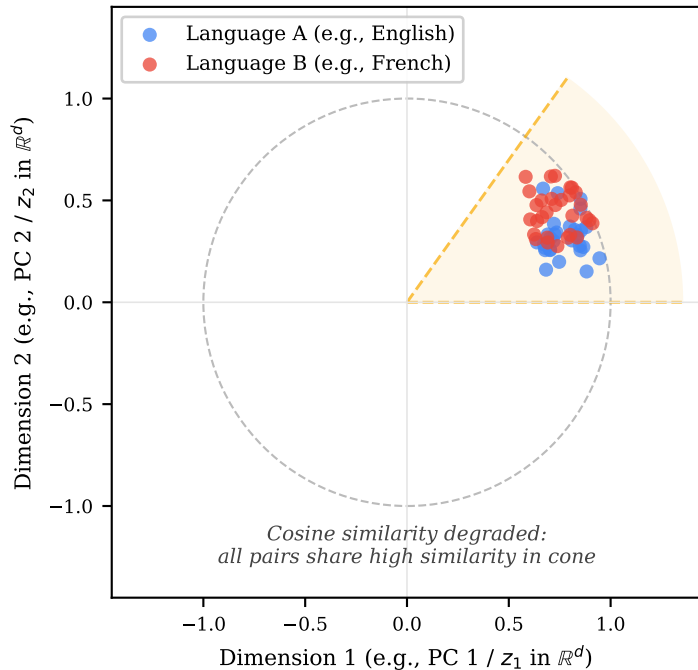
(b) Anisotropic embedding space (LLMs)
