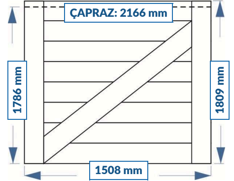
YAN DUVAR GÖRÜNÜMÜ
