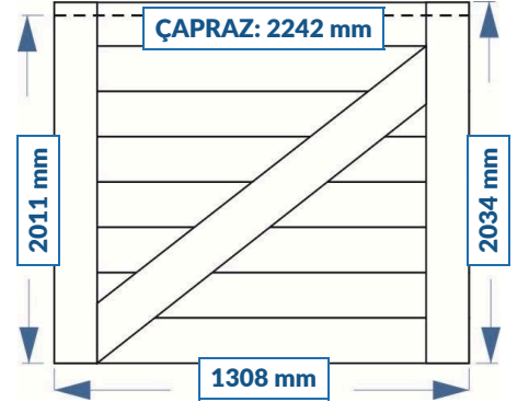
YAN DUVAR GÖRÜNÜMÜ
