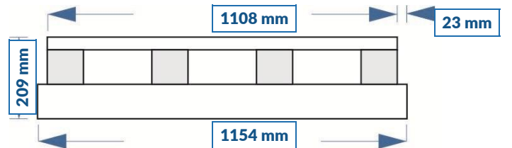
ALT PALET YAN GÖRÜNÜMÜ
