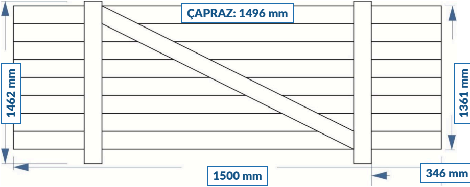
ÖN DUVAR KUŞAK GÖRÜNÜMÜ
