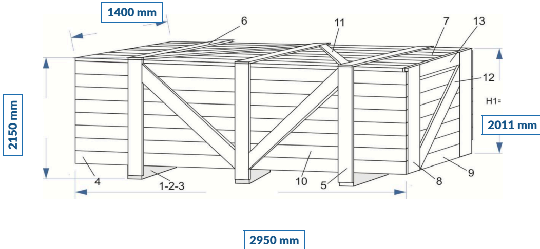
NUMARALI 3B SANDIK MONTAJ GÖRÜNÜMÜ
