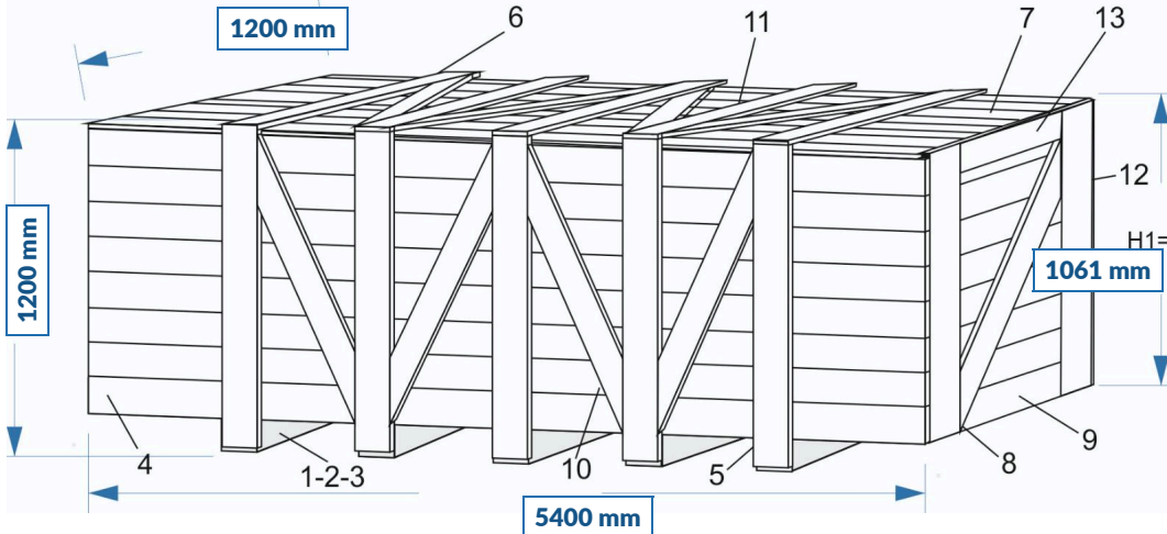
NUMARALI 3B SANDIK MONTAJ GÖRÜNÜMÜ
