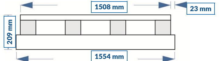
ALT PALET YAN GÖRÜNÜMÜ
