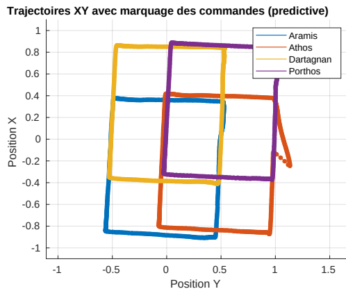
FIGURE 7.17 – Trajectoire des robots avec une perturbation
