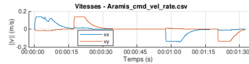
FIGURE 7.11 – Évolution de la vitesse (commande classique)
