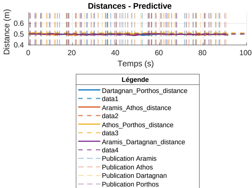
FIGURE 7.16 – Evolution des inter-distances entre les robots
