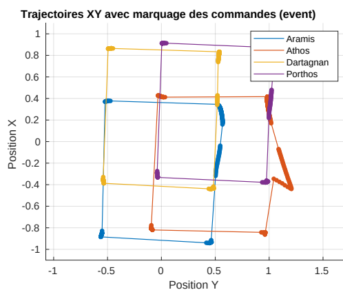
FIGURE 7.12 – Trajectoire des robots avec une perturbation
