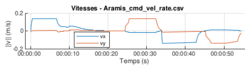
FIGURE 7.10 – Évolution de la vitesse (commande événementielle)
