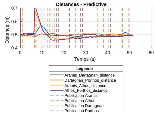
FIGURE 7.18 – Evolution des inter-distances entre les robots avec perturbation
