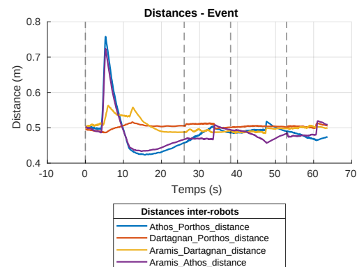
FIGURE 7.13 – Evolution des inter-distances entre les robots avec perturbation
