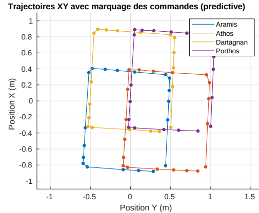
FIGURE 7.15 – Trajectoire de chaque robot de l'essaim
