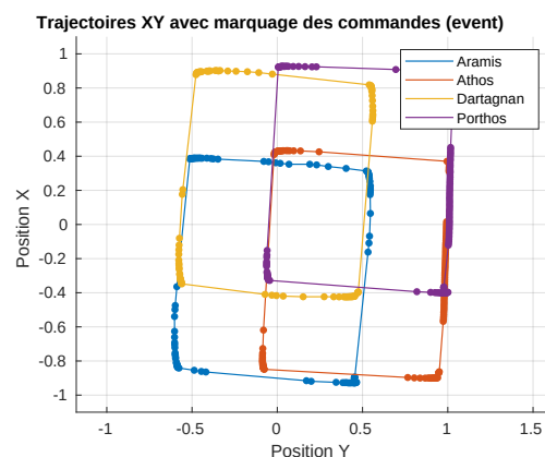
FIGURE 7.8 – Trajectoire de chaque robot de l'essaim
