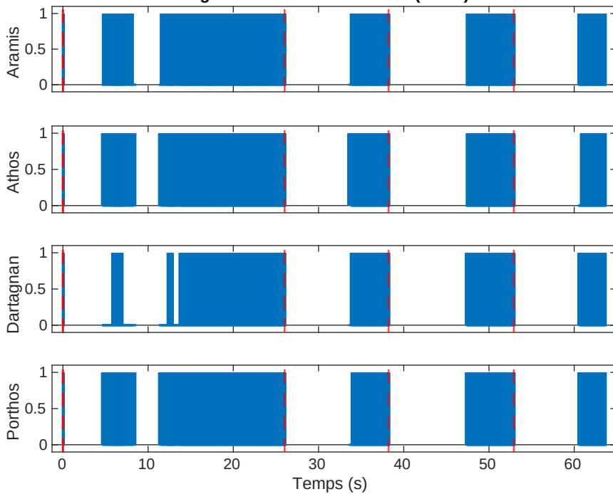
Chronogrammes des commandes (event)
