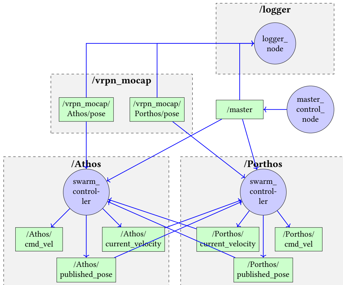
FIGURE 6.3 – Organisation simplifiée du système ROS2 pour la méthode prédictive
