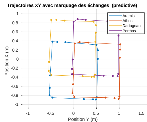
FIGURE 7.16 – Trajectoire de chaque robot de l'essaim
