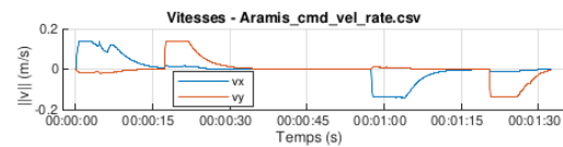
FIGURE 7.12 – Évolution de la vitesse (commande classique)
