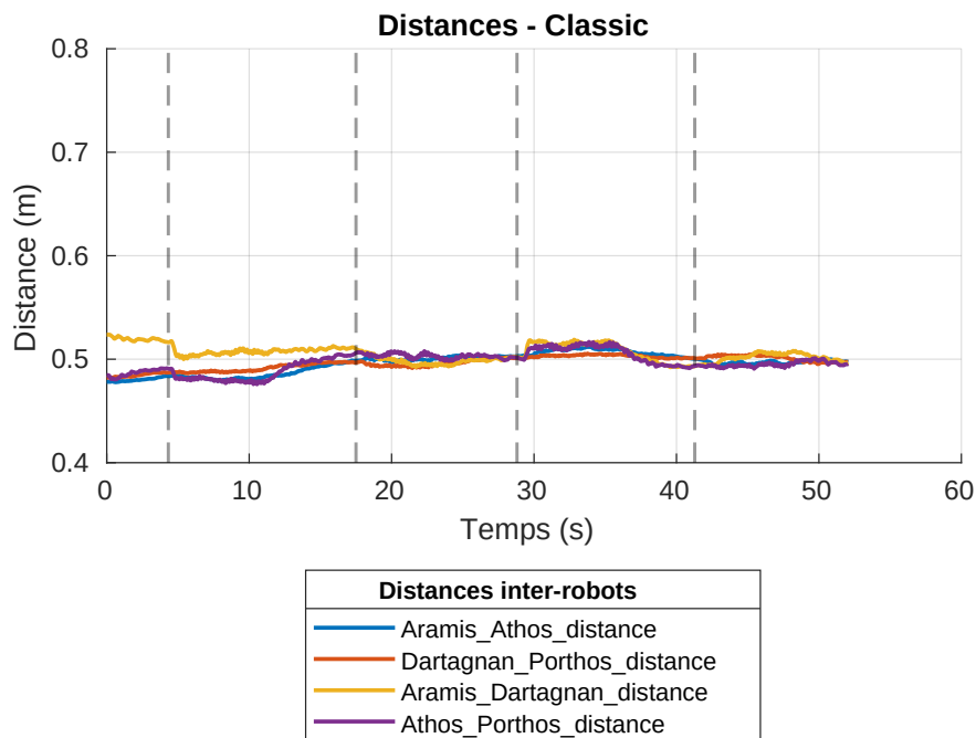
FIGURE 7.4 – Evolution des inter-distances entre les robots
