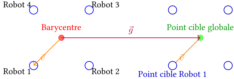
FIGURE 5.1 – Illustration du calcul du point cible individuel à partir du barycentre et du vecteur relatif initial.
