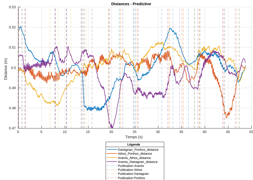
FIGURE 7.17 – Evolution des inter-distances entre les robots
